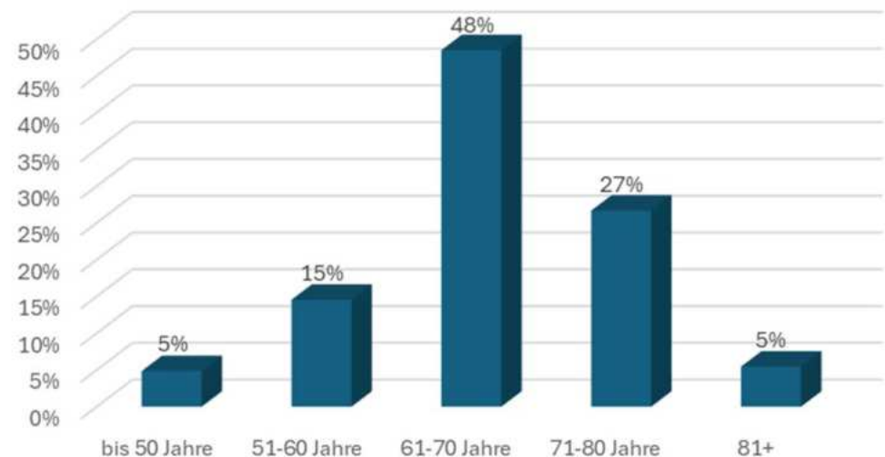
Altersverteilung
